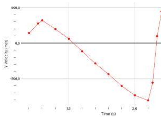
Geschwindigkeit in y – Richtung
